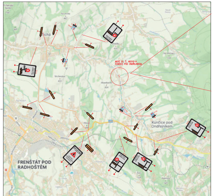
SITUACE PŘECHODNÉHO DOPRAVNÍHO ZNAČENÍ
